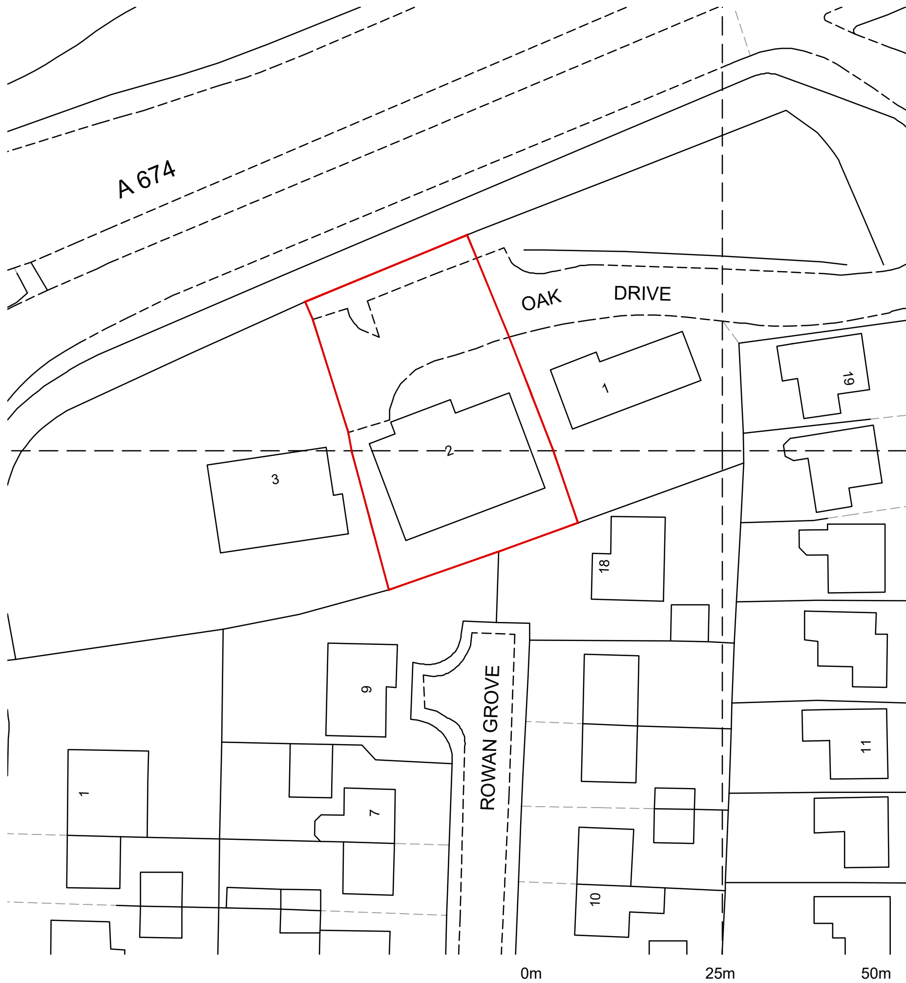
Site Layout 1:500
